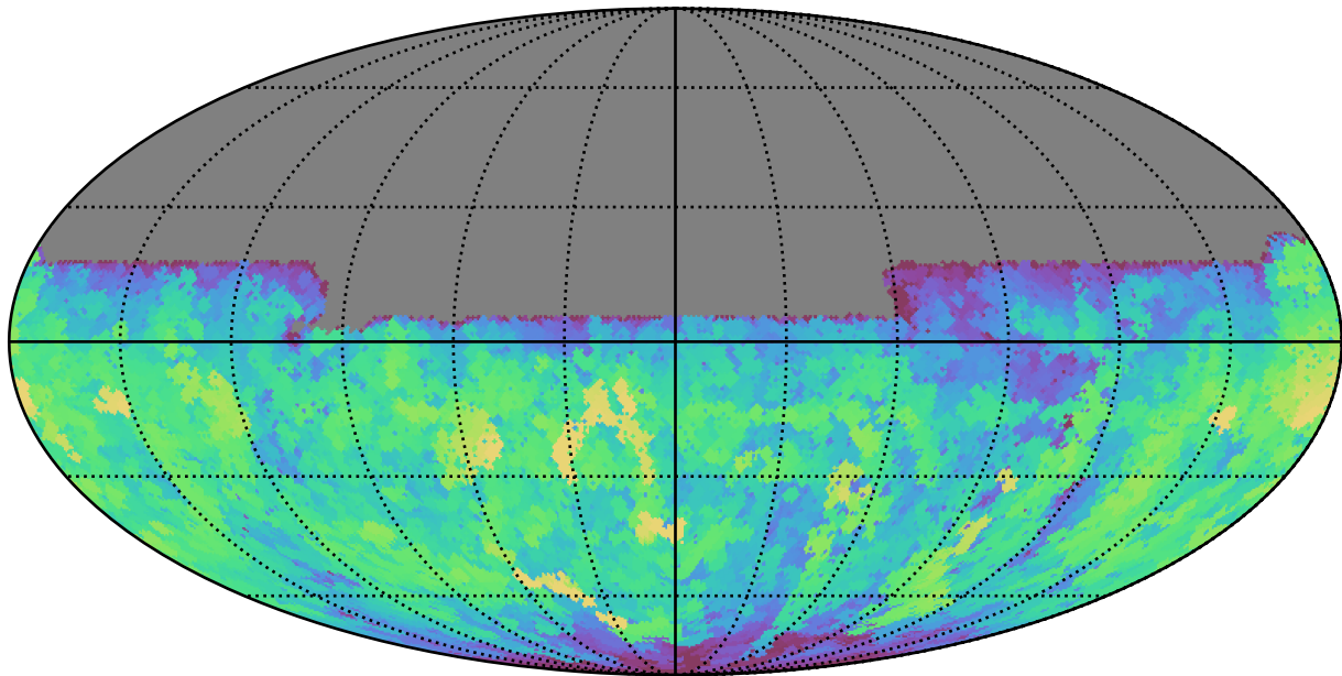
no_magell_roll_v3.4_10yrs All sky u band: Max saturation_mag
