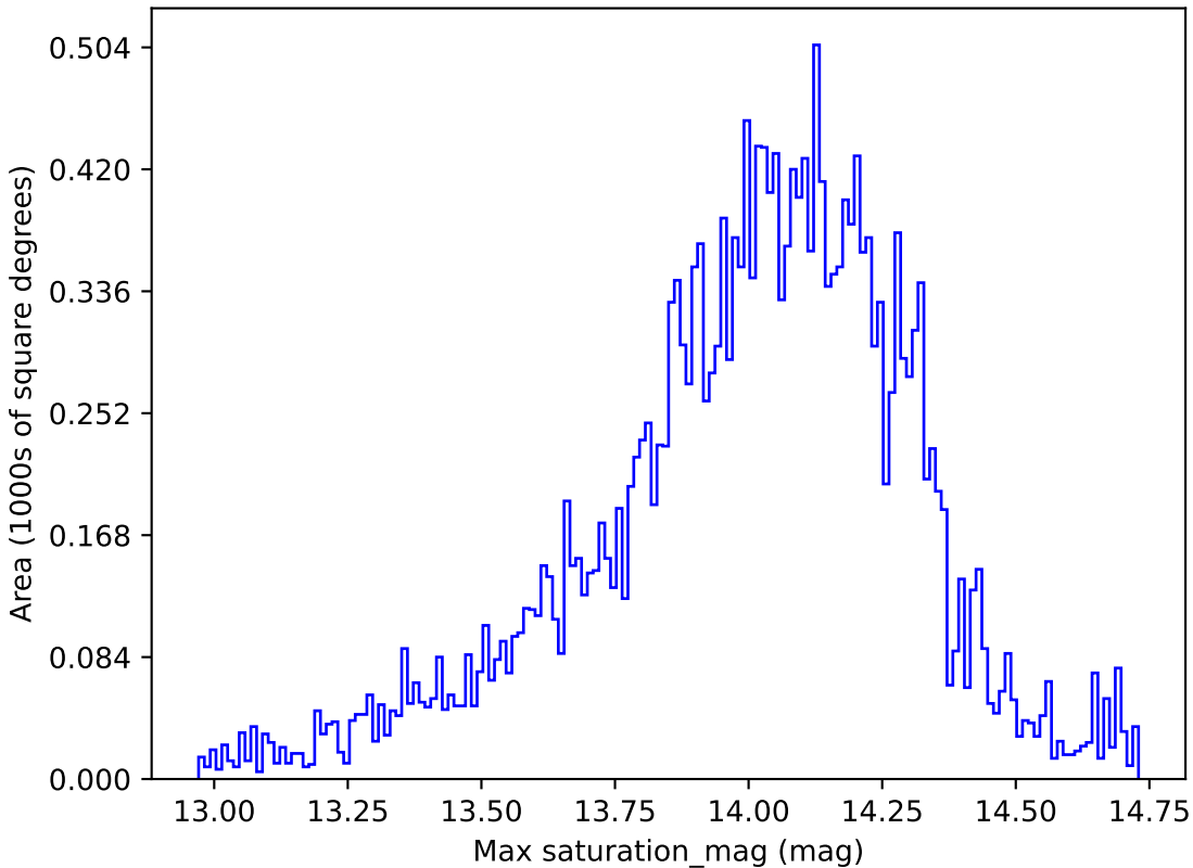
no_magell_roll_v3.4_10yrs All sky u band: Max saturation_mag
