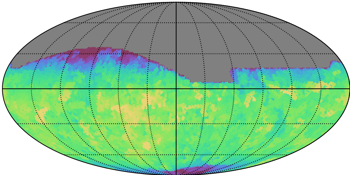
no_magell_roll_v3.4_10yrs All sky r band: Max saturation_mag
