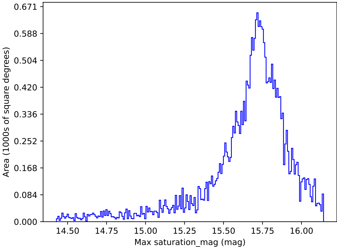
no_magell_roll_v3.4_10yrs All sky r band: Max saturation_mag
