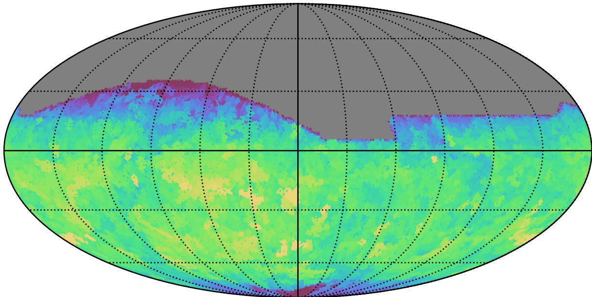
no_magell_roll_v3.4_10yrs All sky i band: Max saturation_mag
