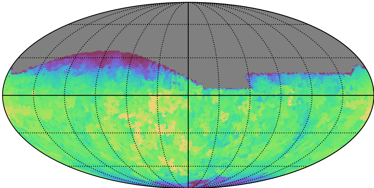
no_magell_roll_v3.4_10yrs All sky g band: Max saturation_mag
