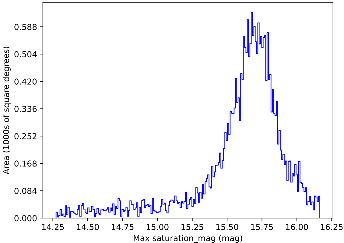
no_magell_roll_v3.4_10yrs All sky g band: Max saturation_mag
