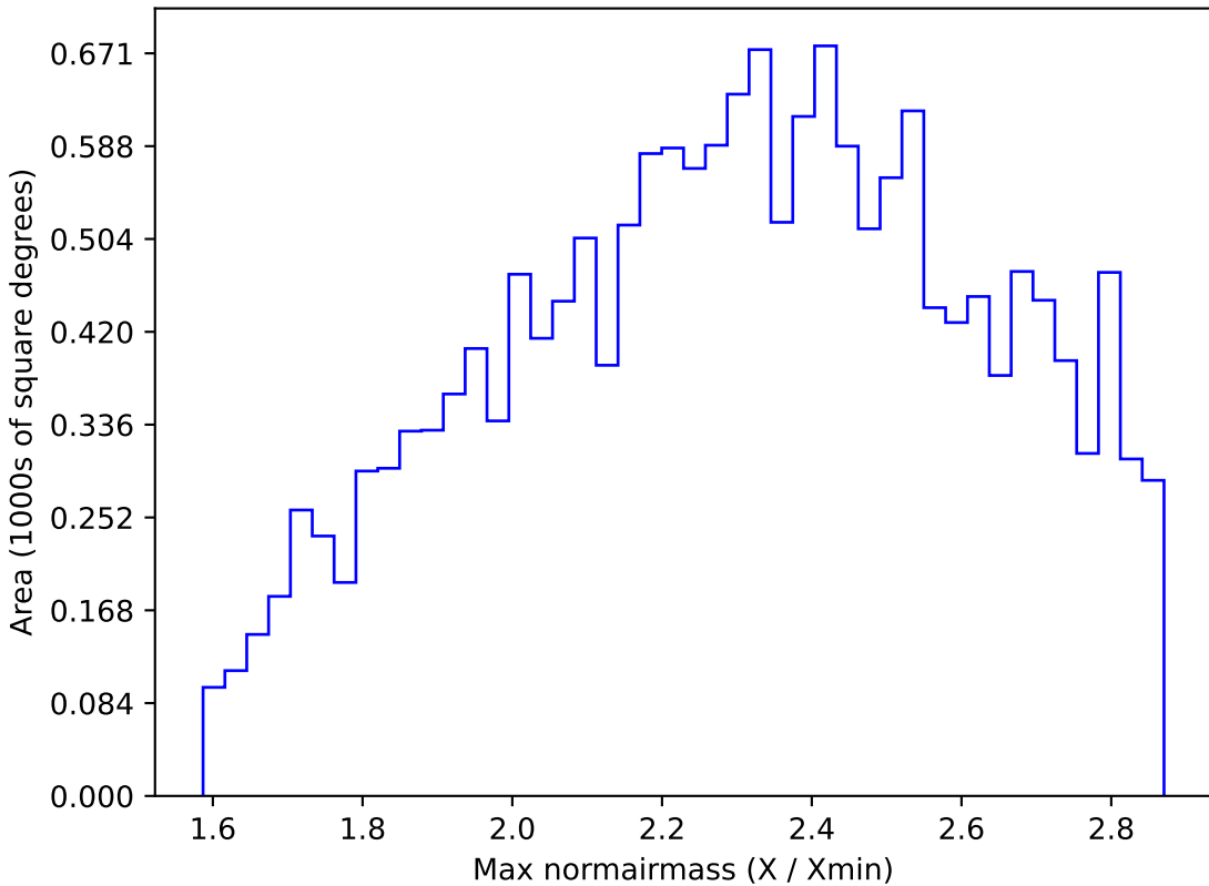
no_magell_roll_v3.4_10yrs WFD z band: Max normairmass
