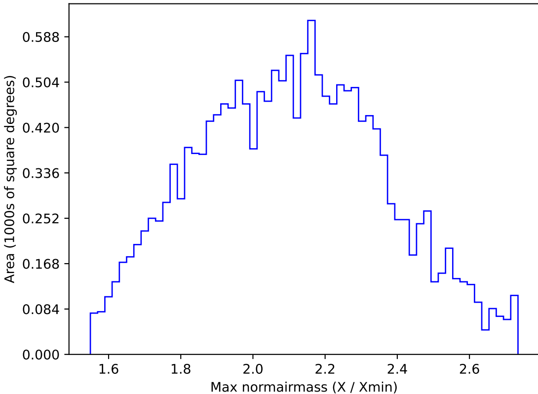
no_magell_roll_v3.4_10yrs WFD y band: Max normairmass
