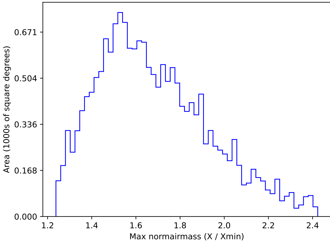
no_magell_roll_v3.4_10yrs WFD u band: Max normairmass
