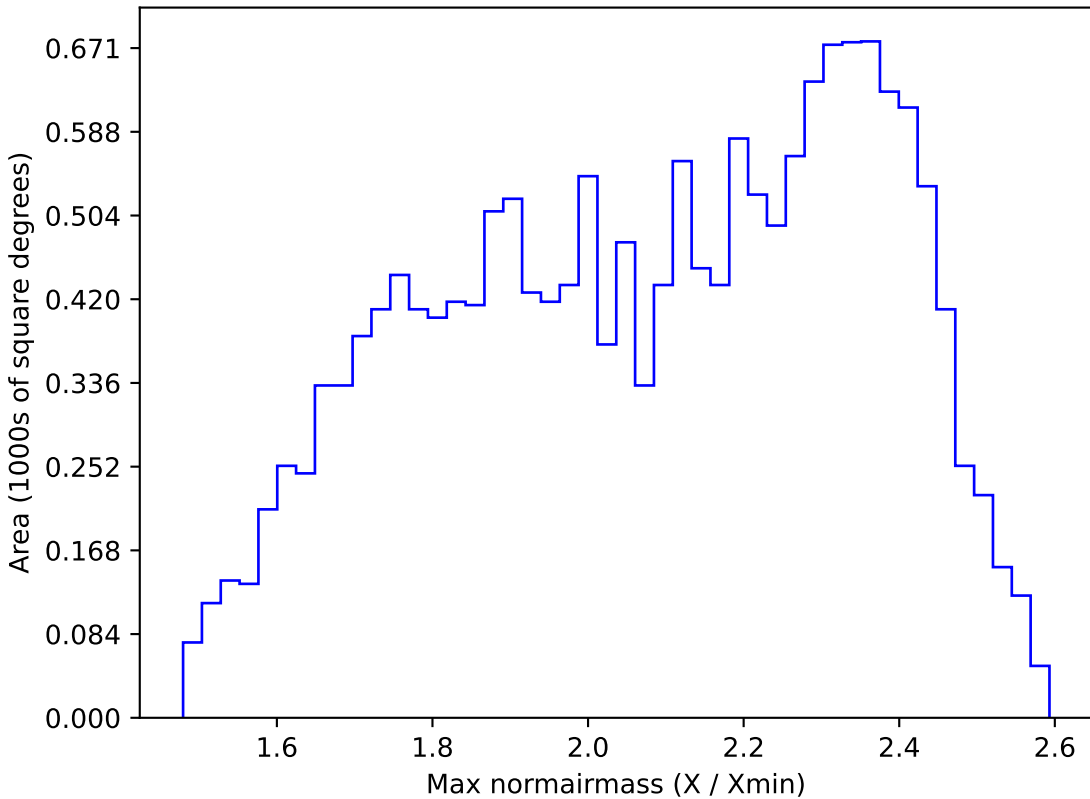
no_magell_roll_v3.4_10yrs WFD r band: Max normairmass
