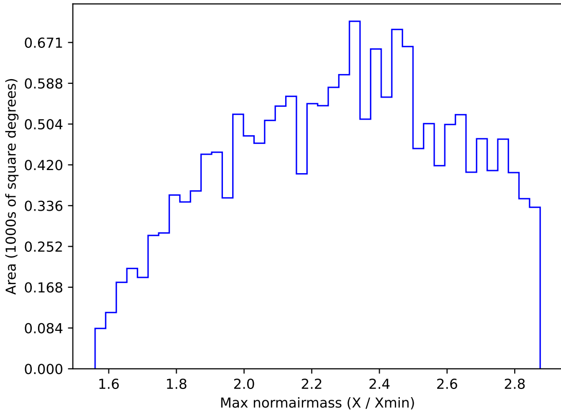
no_magell_roll_v3.4_10yrs WFD i band: Max normairmass
