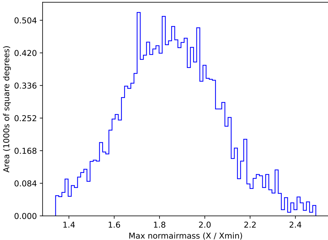
no_magell_roll_v3.4_10yrs WFD g band: Max normairmass
