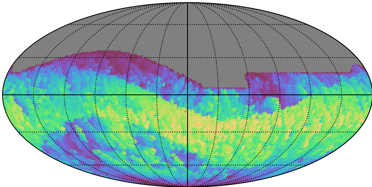
no_magell_roll_v3.4_10yrs All sky z band: Max normairmass
