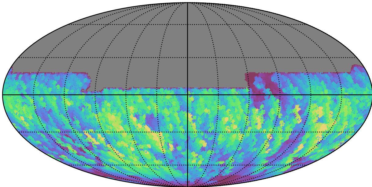
no_magell_roll_v3.4_10yrs All sky y band: Max normairmass
