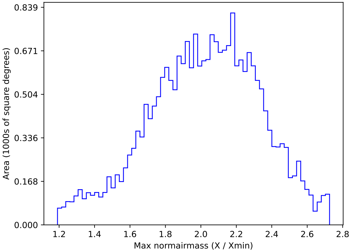
no_magell_roll_v3.4_10yrs All sky y band: Max normairmass
