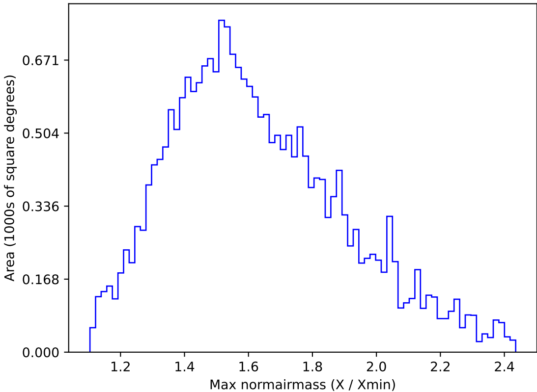
no_magell_roll_v3.4_10yrs All sky u band: Max normairmass
