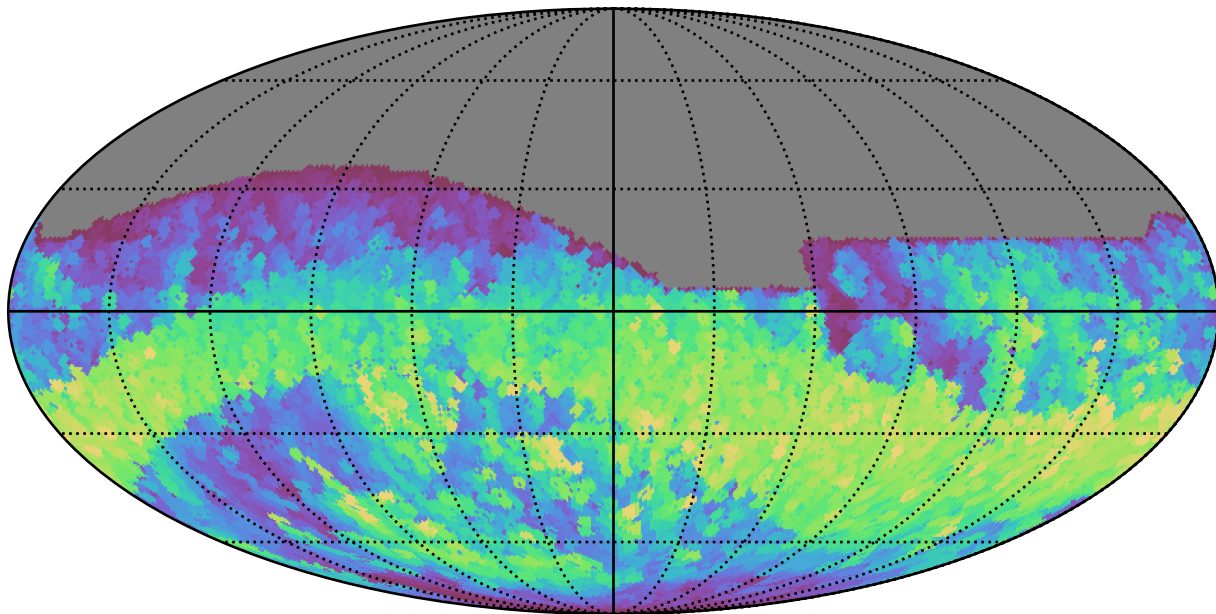
no_magell_roll_v3.4_10yrs All sky r band: Max normairmass
