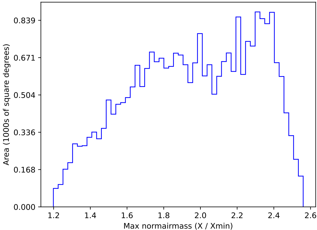
no_magell_roll_v3.4_10yrs All sky r band: Max normairmass
