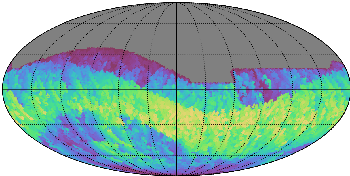
no_magell_roll_v3.4_10yrs All sky i band: Max normairmass
