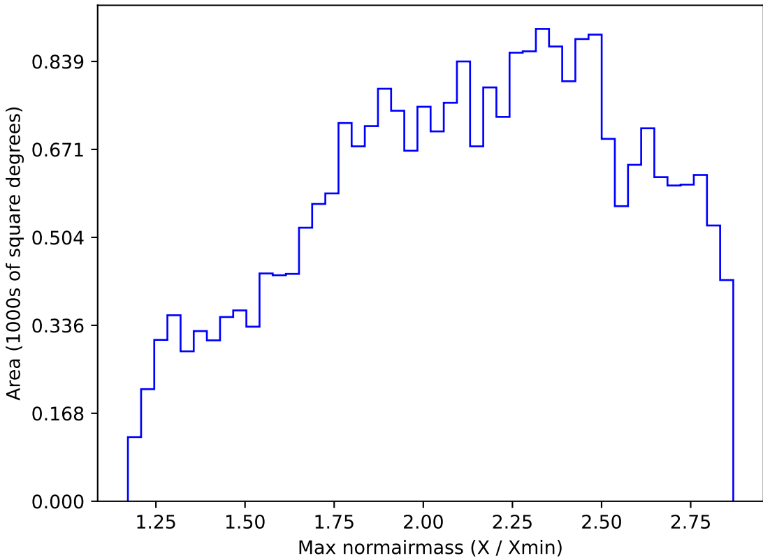
no_magell_roll_v3.4_10yrs All sky i band: Max normairmass
