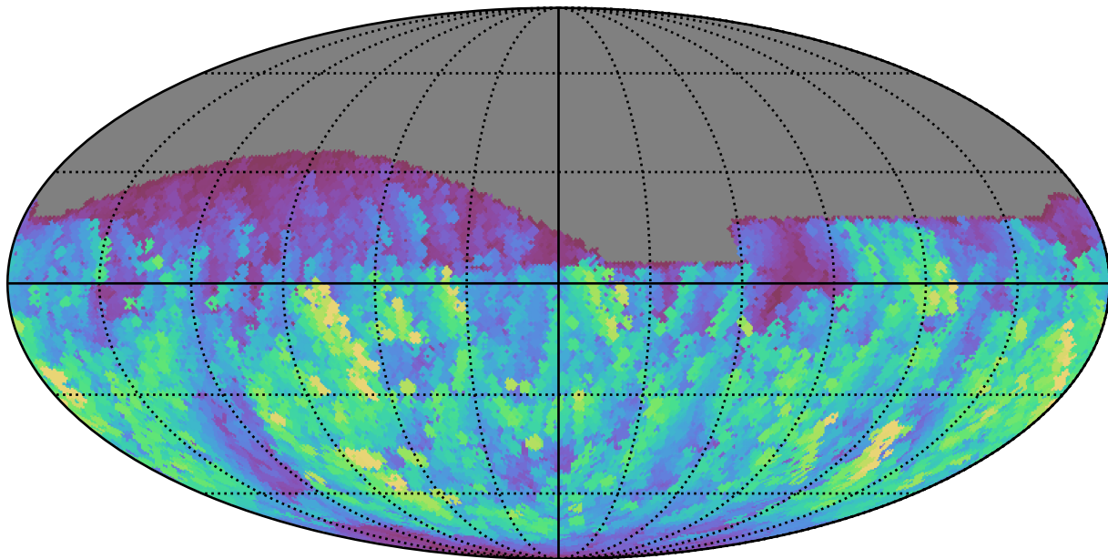
no_magell_roll_v3.4_10yrs All sky g band: Max normairmass
