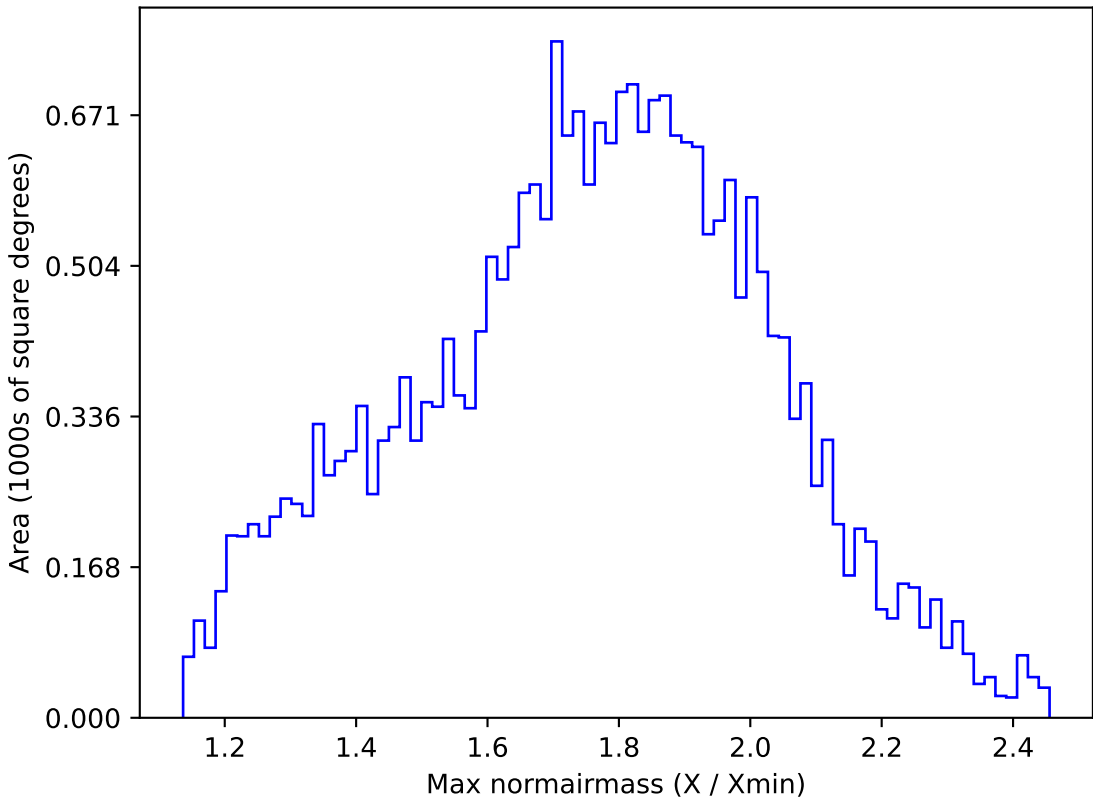
no_magell_roll_v3.4_10yrs All sky g band: Max normairmass
