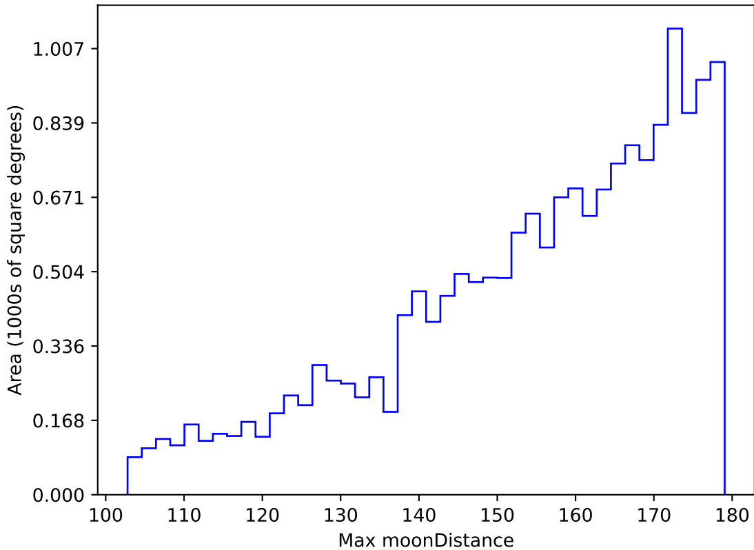
no_magell_roll_v3.4_10yrs WFD z band: Max moonDistance
