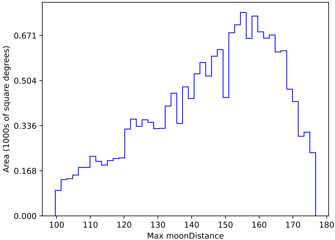
no_magell_roll_v3.4_10yrs WFD y band: Max moonDistance
