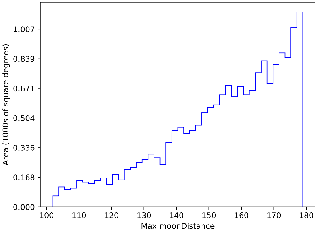
no_magell_roll_v3.4_10yrs WFD u band: Max moonDistance
