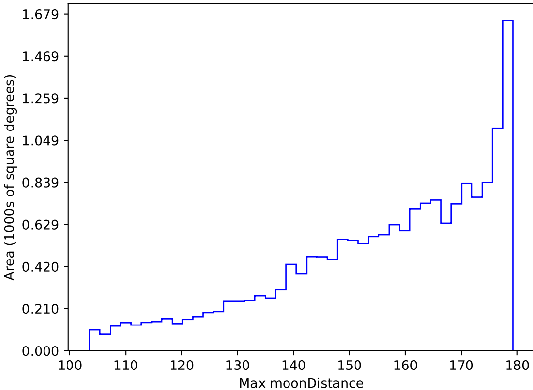
no_magell_roll_v3.4_10yrs WFD r band: Max moonDistance
