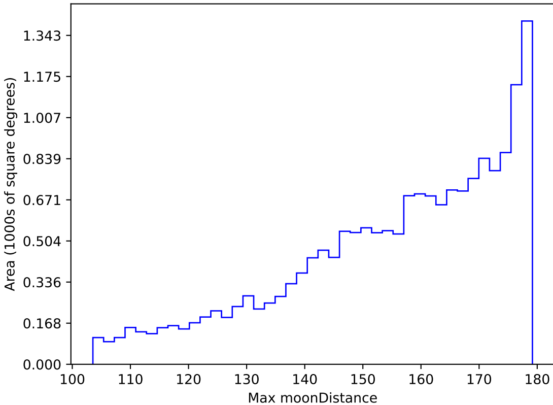
no_magell_roll_v3.4_10yrs WFD i band: Max moonDistance
