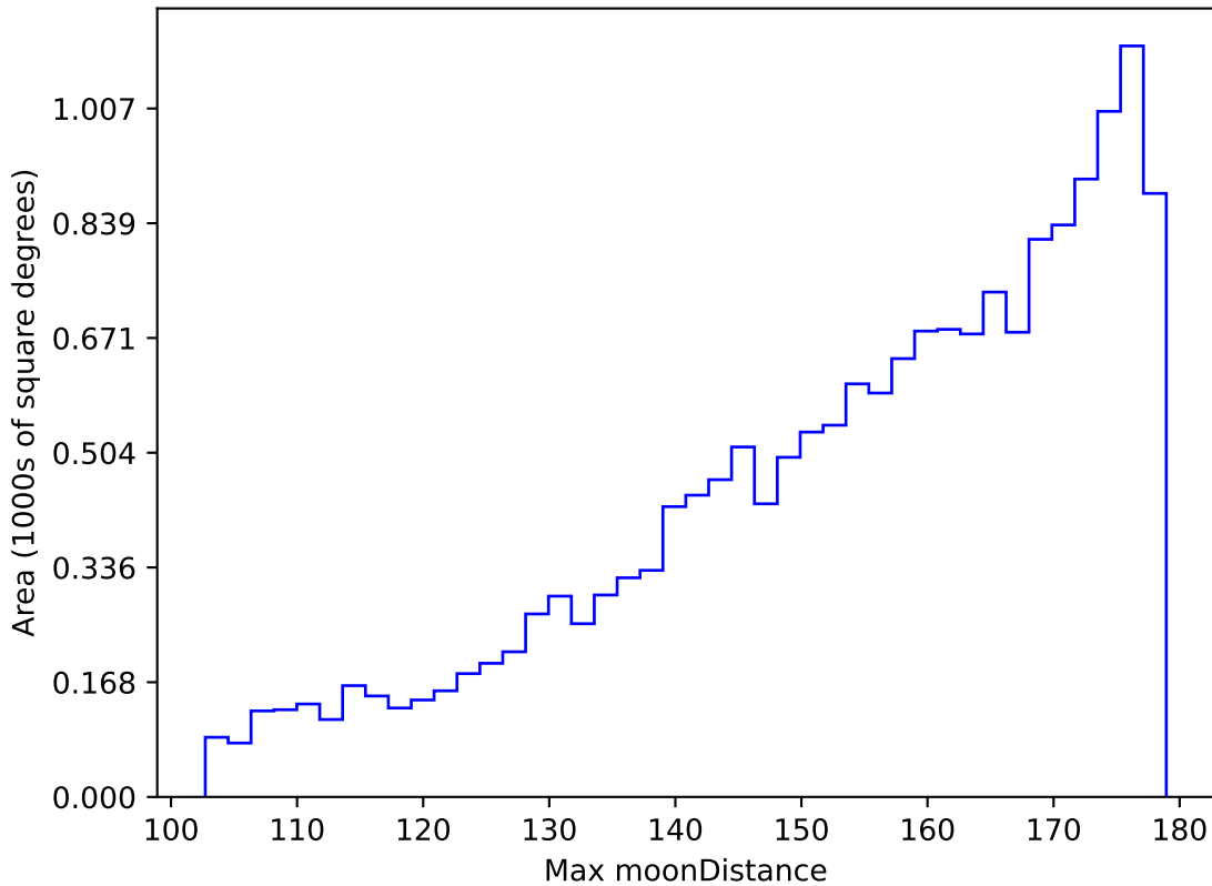
no_magell_roll_v3.4_10yrs WFD g band: Max moonDistance
