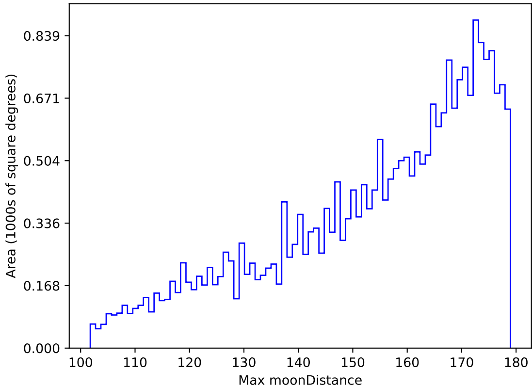
no_magell_roll_v3.4_10yrs All sky z band: Max moonDistance
