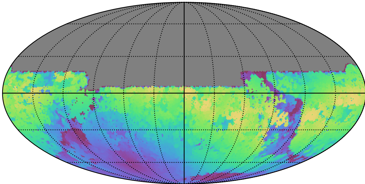
no_magell_roll_v3.4_10yrs All sky y band: Max moonDistance
