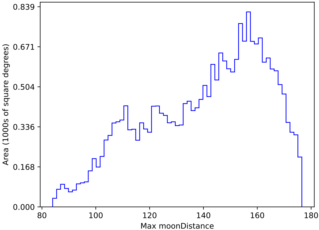
no_magell_roll_v3.4_10yrs All sky y band: Max moonDistance
