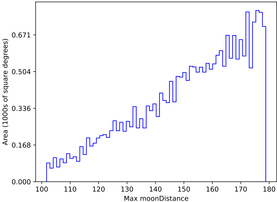
no_magell_roll_v3.4_10yrs All sky u band: Max moonDistance
