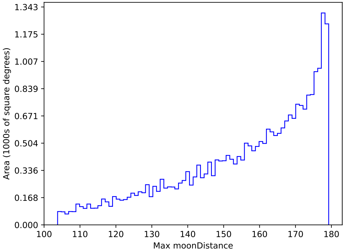
no_magell_roll_v3.4_10yrs All sky r band: Max moonDistance
