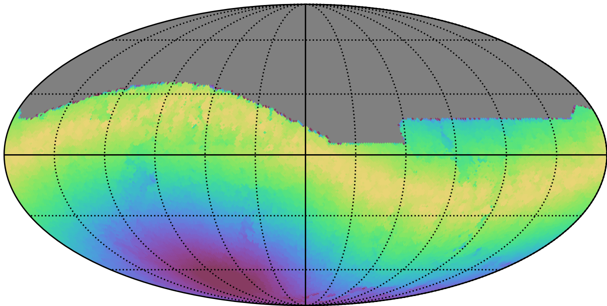
no_magell_roll_v3.4_10yrs All sky i band: Max moonDistance
