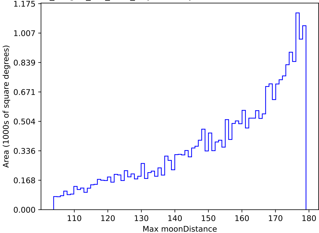
no_magell_roll_v3.4_10yrs All sky i band: Max moonDistance
