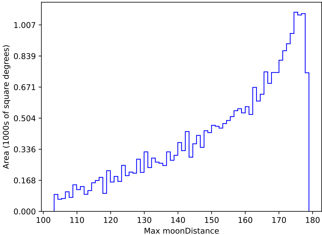
no_magell_roll_v3.4_10yrs All sky g band: Max moonDistance
