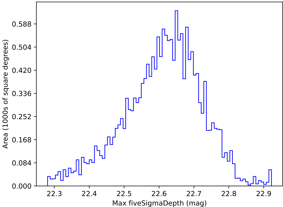
no_magell_roll_v3.4_10yrs WFD y band: Max fiveSigmaDepth
