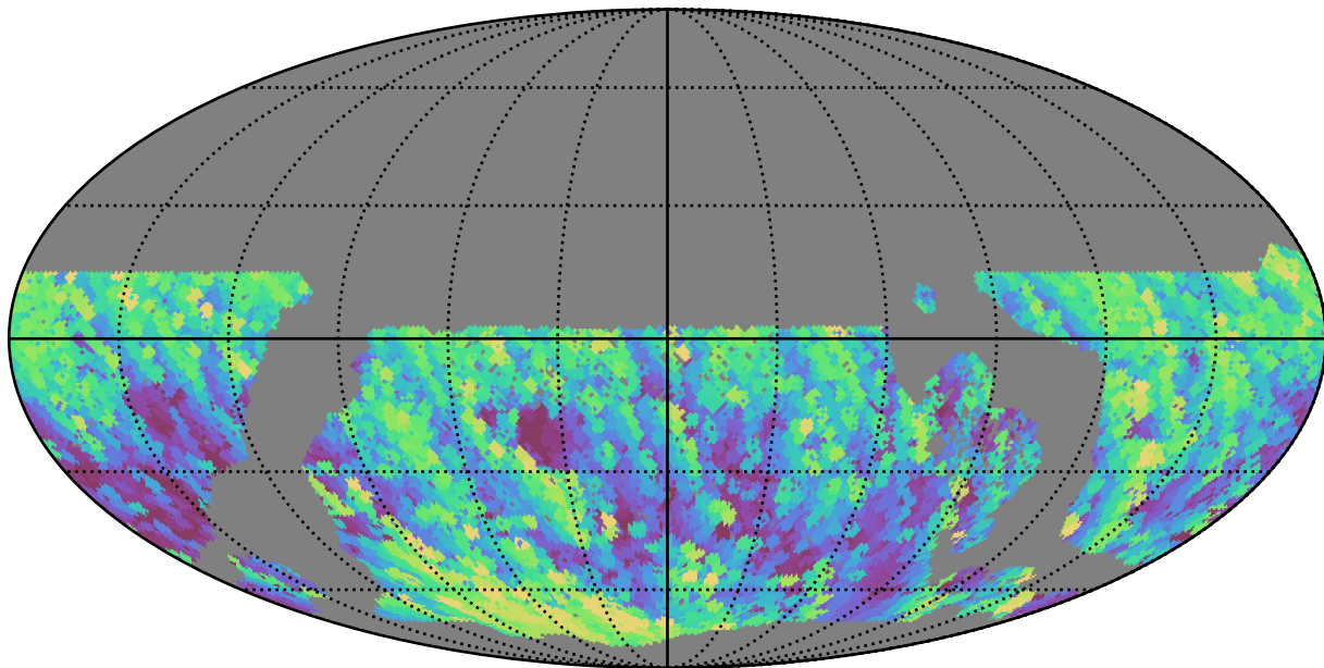
no_magell_roll_v3.4_10yrs WFD y band: Max airmass
