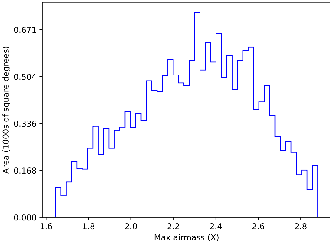
no_magell_roll_v3.4_10yrs WFD y band: Max airmass
