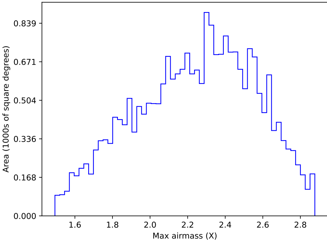
no_magell_roll_v3.4_10yrs All sky y band: Max airmass
