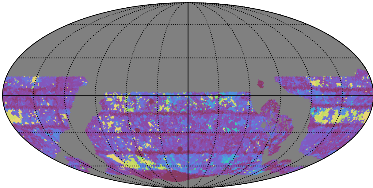
no_magell_roll_v3.4_10yrs WFD y band: Max Inter-Night Gap
