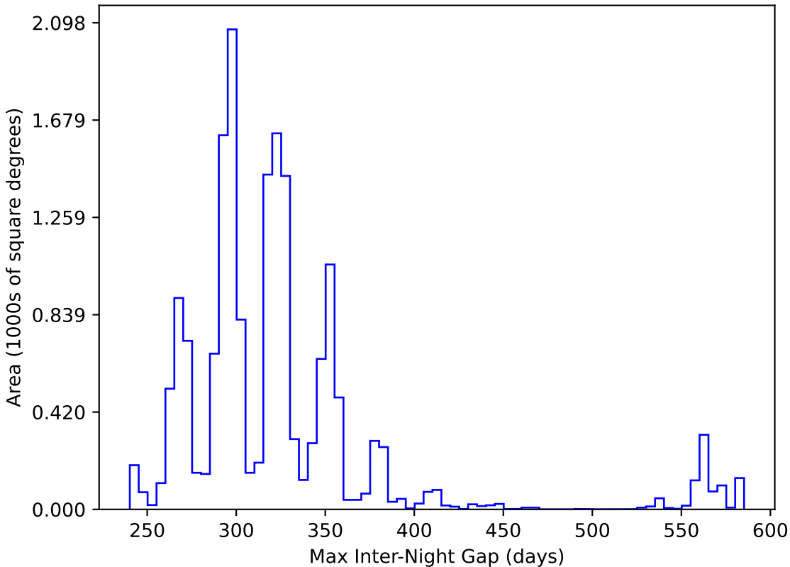
no_magell_roll_v3.4_10yrs WFD y band: Max Inter-Night Gap
