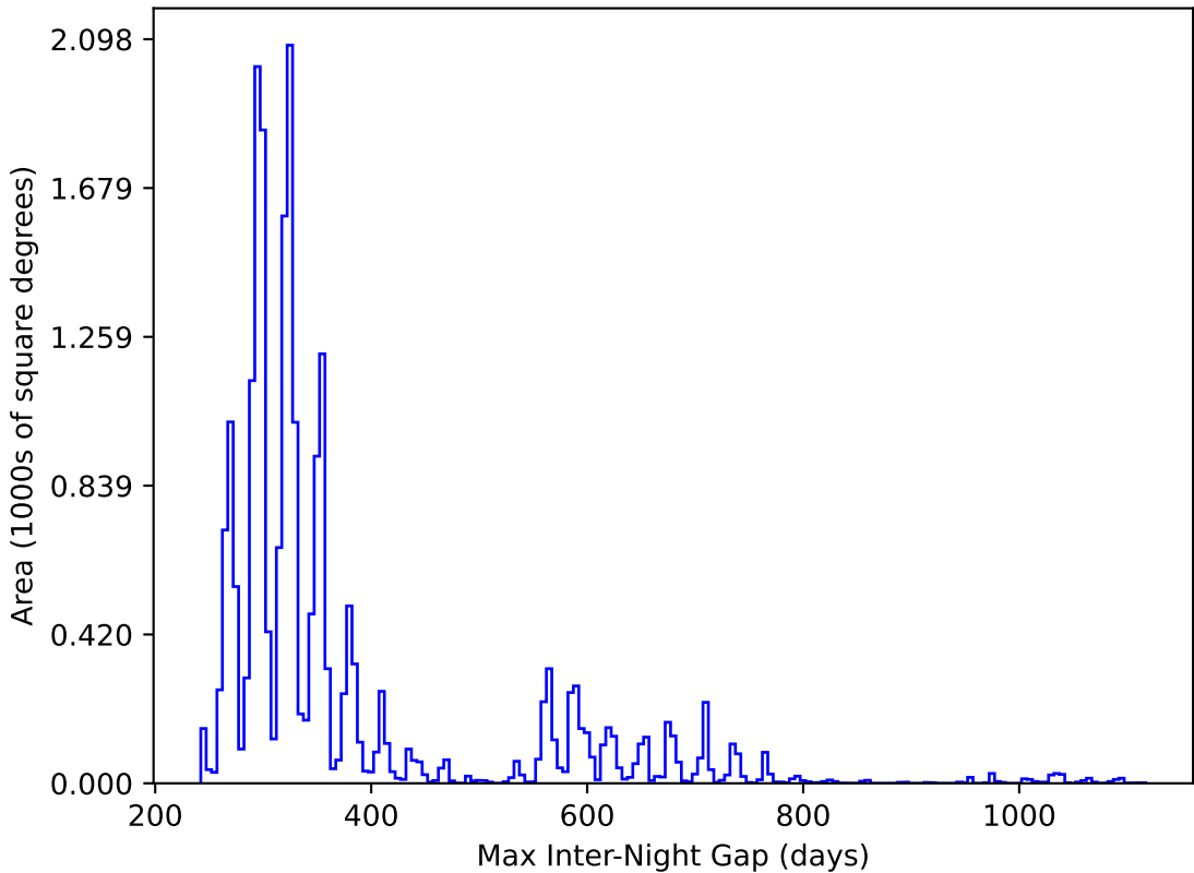
no_magell_roll_v3.4_10yrs All sky y band: Max Inter-Night Gap
