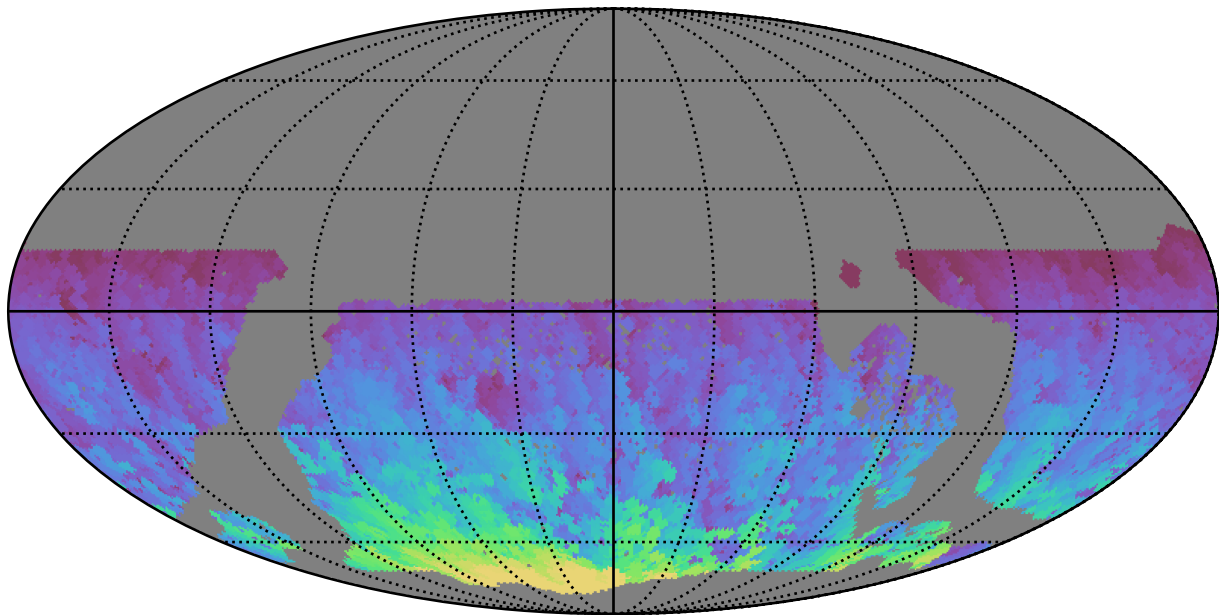
no_magell_roll_v3.4_10yrs WFD y band: Max HA
