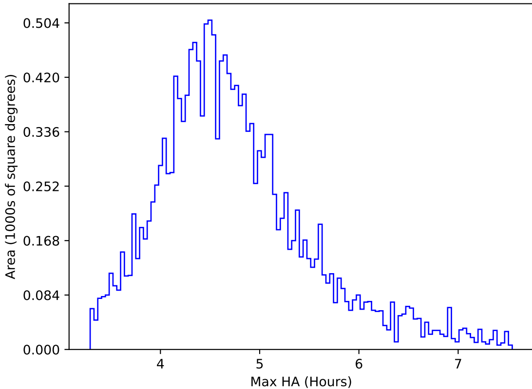
no_magell_roll_v3.4_10yrs WFD y band: Max HA
