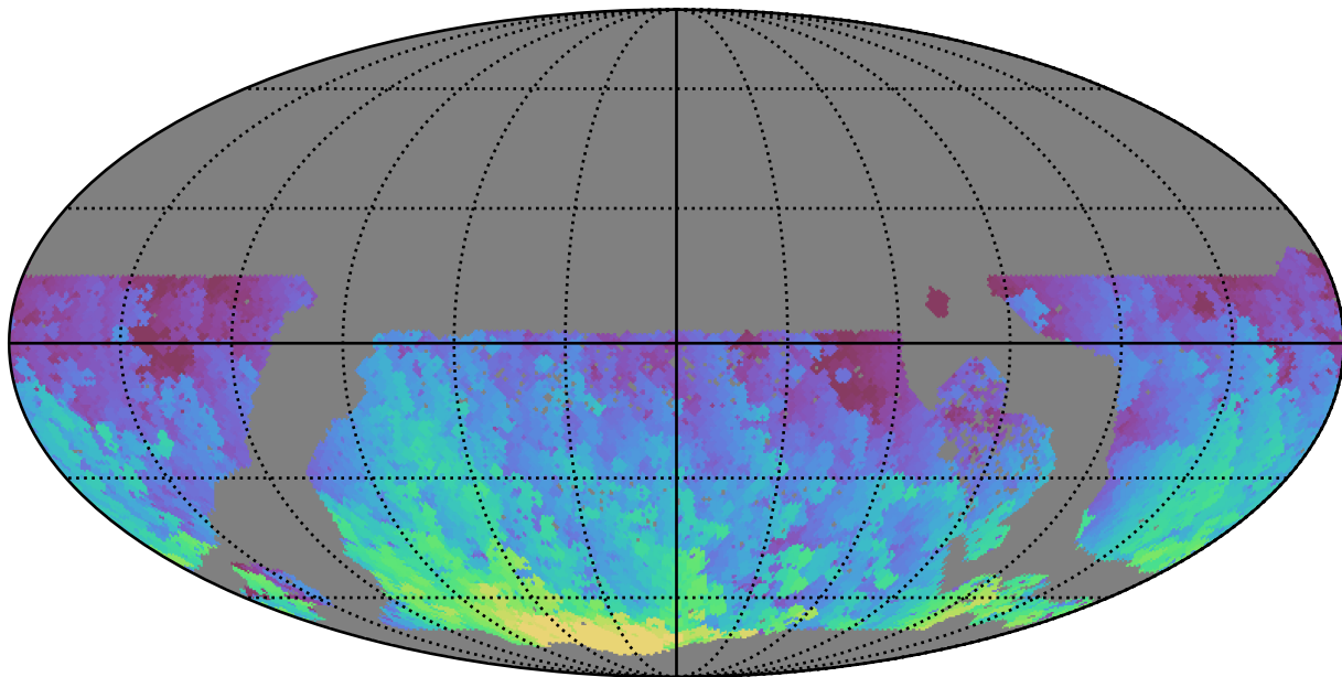
no_magell_roll_v3.4_10yrs WFD u band: Max HA
