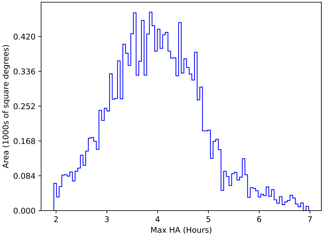
no_magell_roll_v3.4_10yrs WFD u band: Max HA
