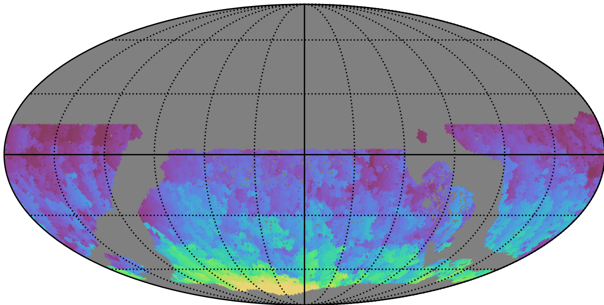
no_magell_roll_v3.4_10yrs WFD r band: Max HA
