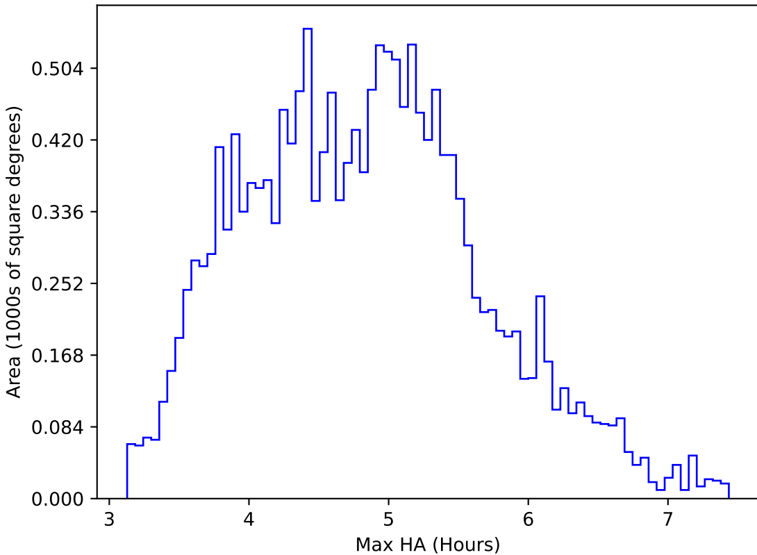
no_magell_roll_v3.4_10yrs WFD i band: Max HA
